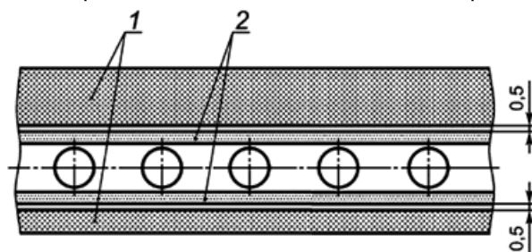
Рисунок 4 - Пригодная толщина обкладок стандартной ленты
